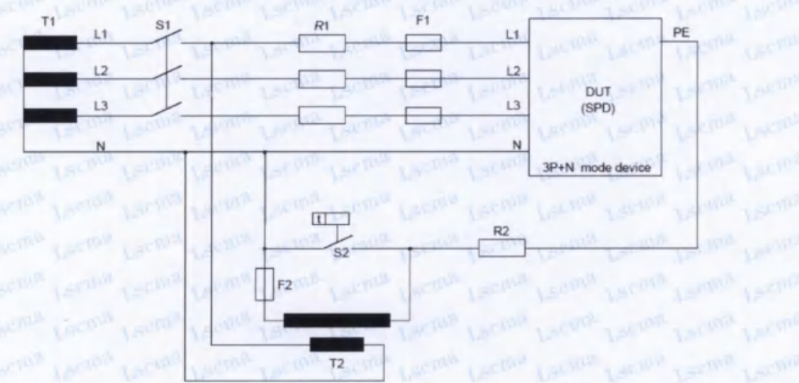
高（中）压系统的故障引起的暂时过电压（TOV）下试验等效电路图
