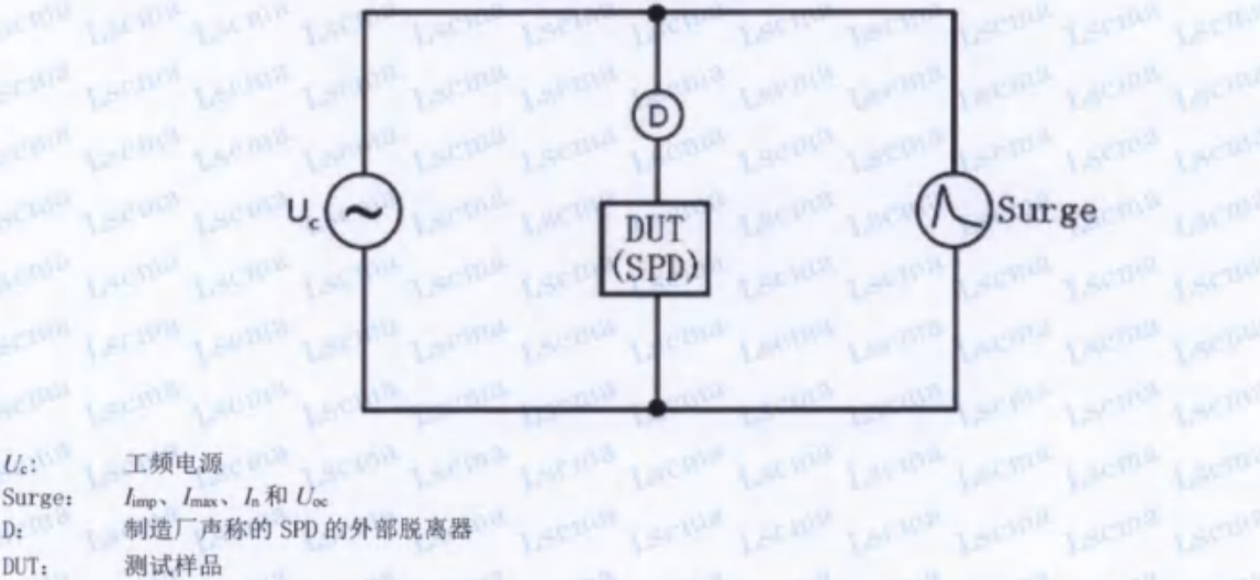
高（中）压系统的故障引起的暂时过电压（TOV）下试验等效电路图
