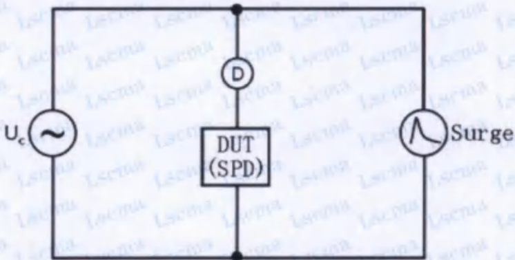
动作负载的测试设置
